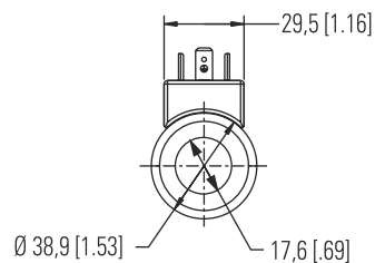
G0 DIN 43650-A Connector
