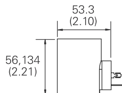
"G" - DIN 43650
