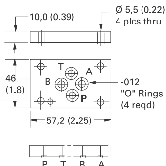
Spacer plate 02-185273
